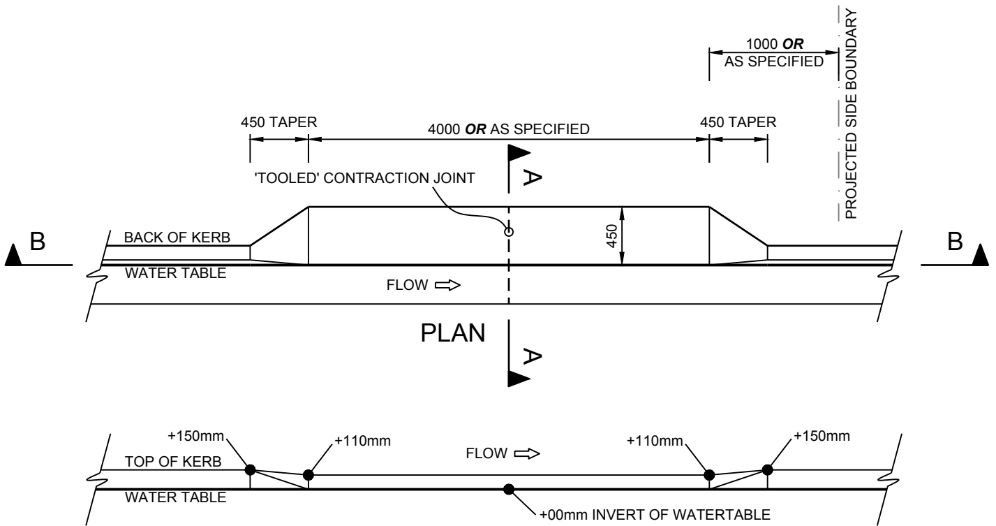
ELEVATION B-B
