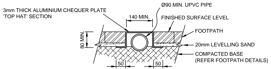
SECTION A-A
